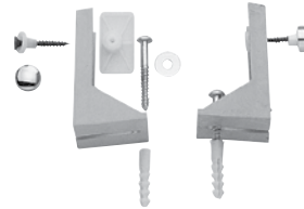
733 € 2,60 Coppia zanche in plastica antiurto a L con viti, per fissaggio laterale W.C. e bidet. Couple wall brackets in plastic, shock-resistant, L shaped, with screws, for side WC and bidet fixing.
