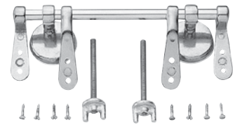
747 € 12,00 Coppia cerniere per sedile WC, in ottone cromato, tipo con tubetto per sedili in legno, con 8 viti in ottone. Couple hinges for WC seat, in C.P. brass, kind with pipe for wooden seats, with 8 brass screws.
