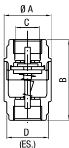
383 Valvola di ritegno STAR. STAR check valve.
