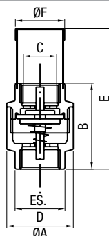
381 Valvola di fondo, con filtro. REMER foot valve, with filter.
