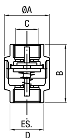
380 Valvola di ritegno. REMER check valve.
